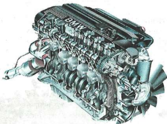
двигатель внутреннего сгорания
